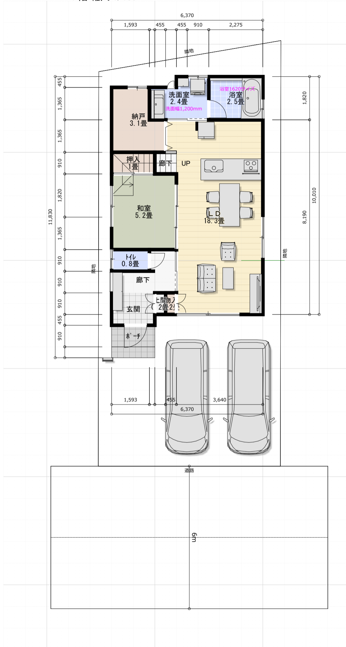
1階 縮尺 1/100
