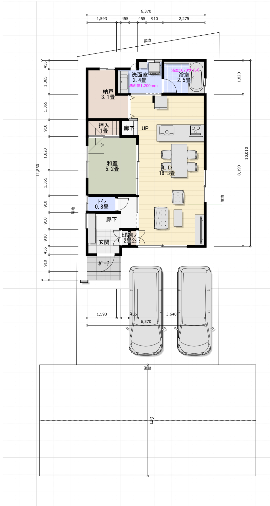
1階 縮尺 1/100
