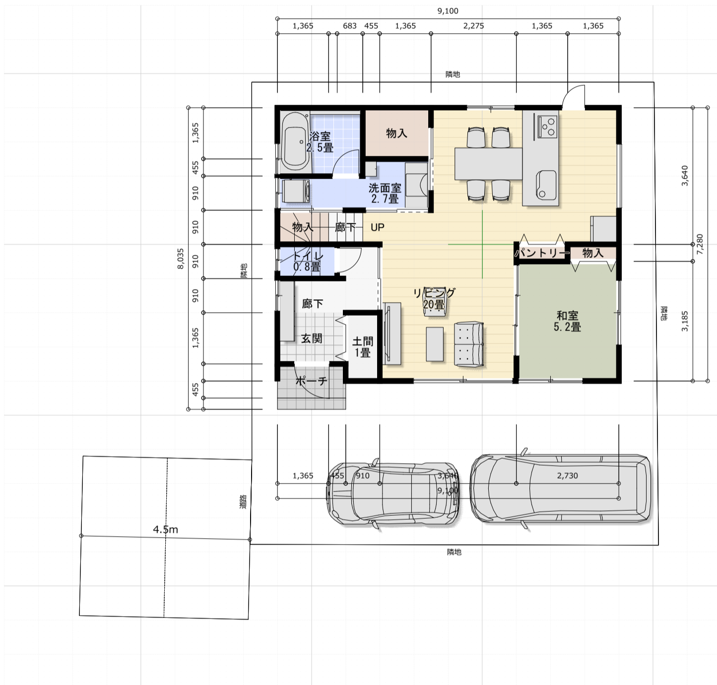
1階 縮尺 1/100
